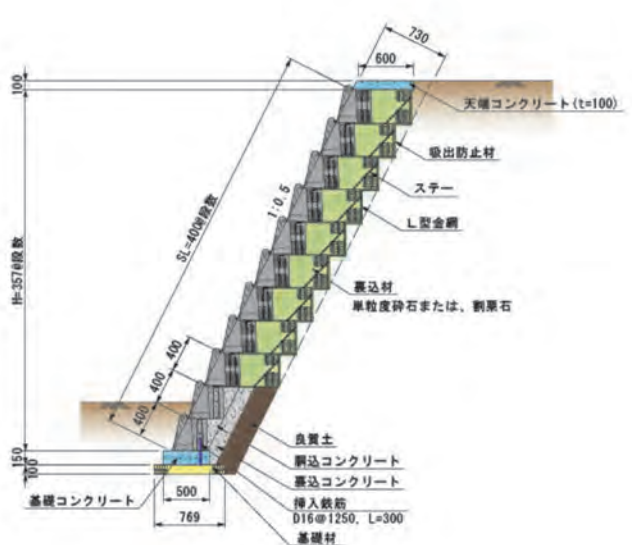
道路擁壁 空積 (500型 控 73cm)
