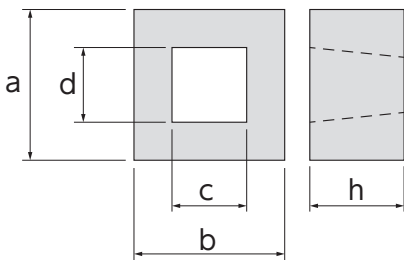
規格図
