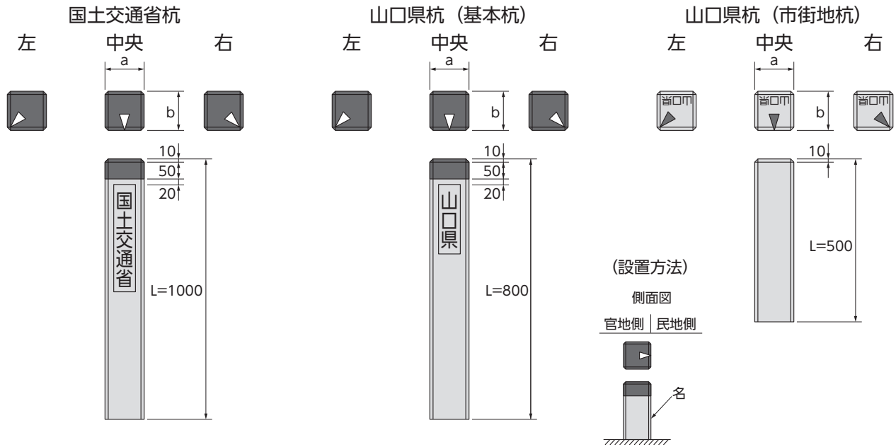
規格表
